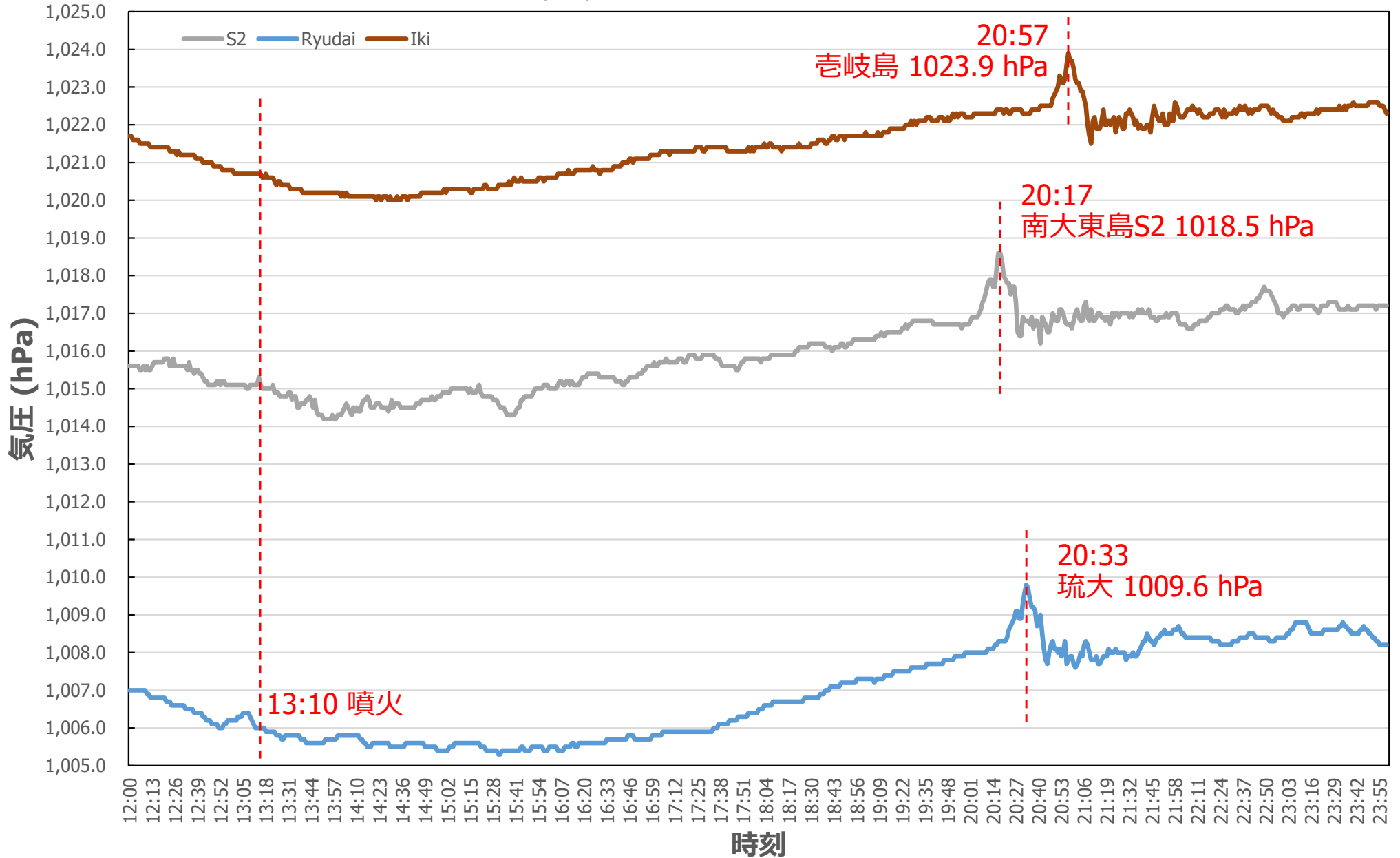
2022/01/15 各地気圧センサー推移
